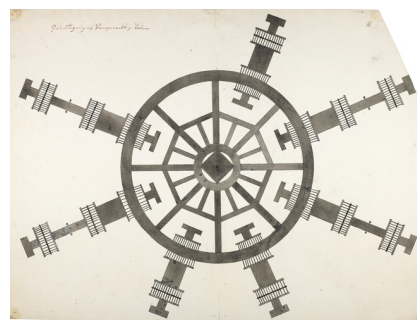
2) Johannes Wiedewelt: Skitse til relief på Henrik Gerners Monument 1789, 44,4 x 59,9 cm, tusch og vandfarve. Bet: "Grundtegnning af Pumpeværket i Doken". KBSA.
